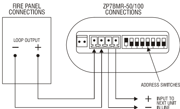
ZP7BMR ADDRESSABLE WIRING
